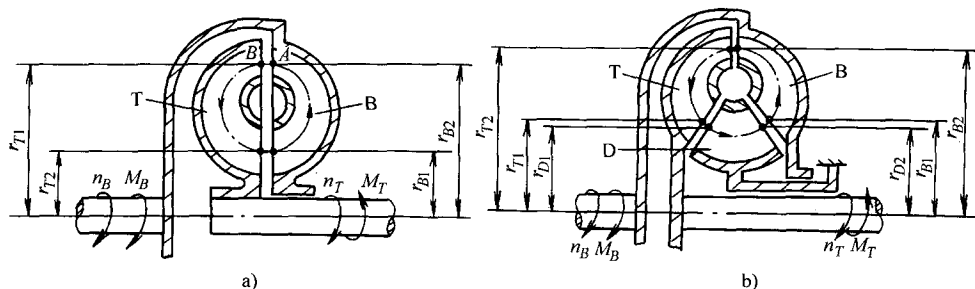
图 25.1-1 液力元件原理简图
