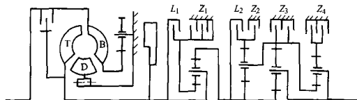
图 25.1-2 CLBT5861 液力传动装置传动简图
