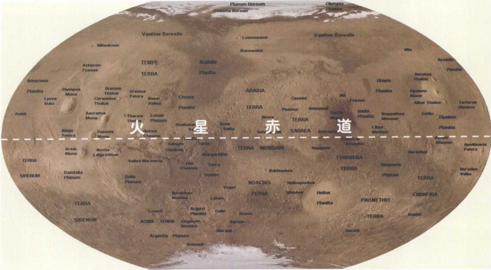
彩色插图七十二 火星全球地图，赤道沿线是最有可能找到水火山口的地区
