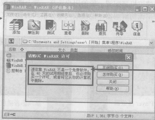
图 1-3 WinRAR 3.62 试用版
