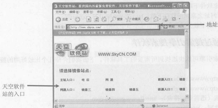
图 1-7 天空软件站
