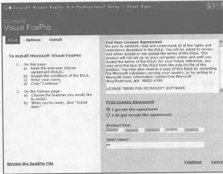
图 1—3 输入产品序列号和用户名对话框
