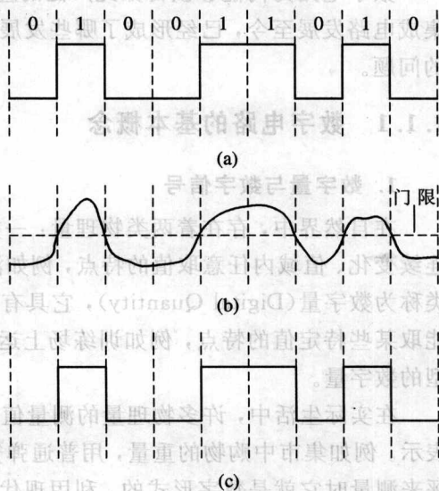
图1-2 数字电路对接收信号整形
