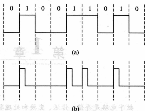
图1-1 数字信号的传输波形
