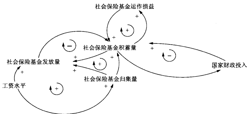
图 2 因果关系图
