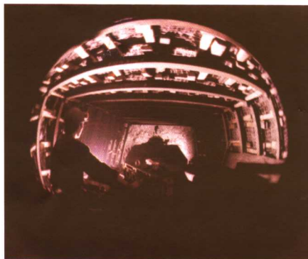
综合机械化掘进迎头
