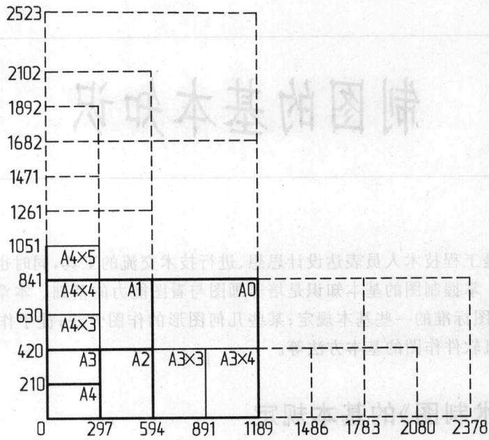
图 1-1 图纸幅面
