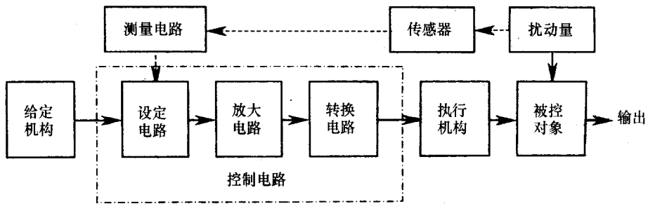
图 1-8 开环控制系统的基本组成
