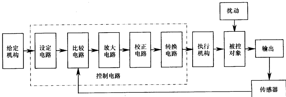
图 1-9 闭环控制系统的基本组成
