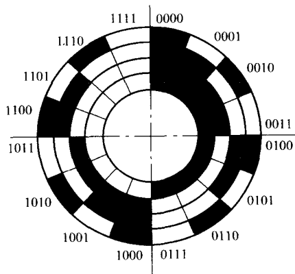
图 1-5 码盘
