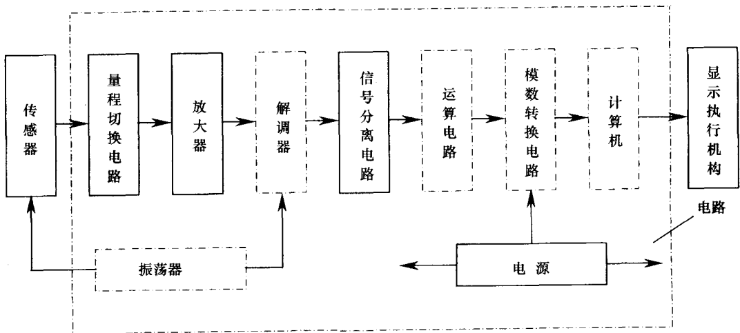
图 1-6 模拟式测量电路的基本组成
