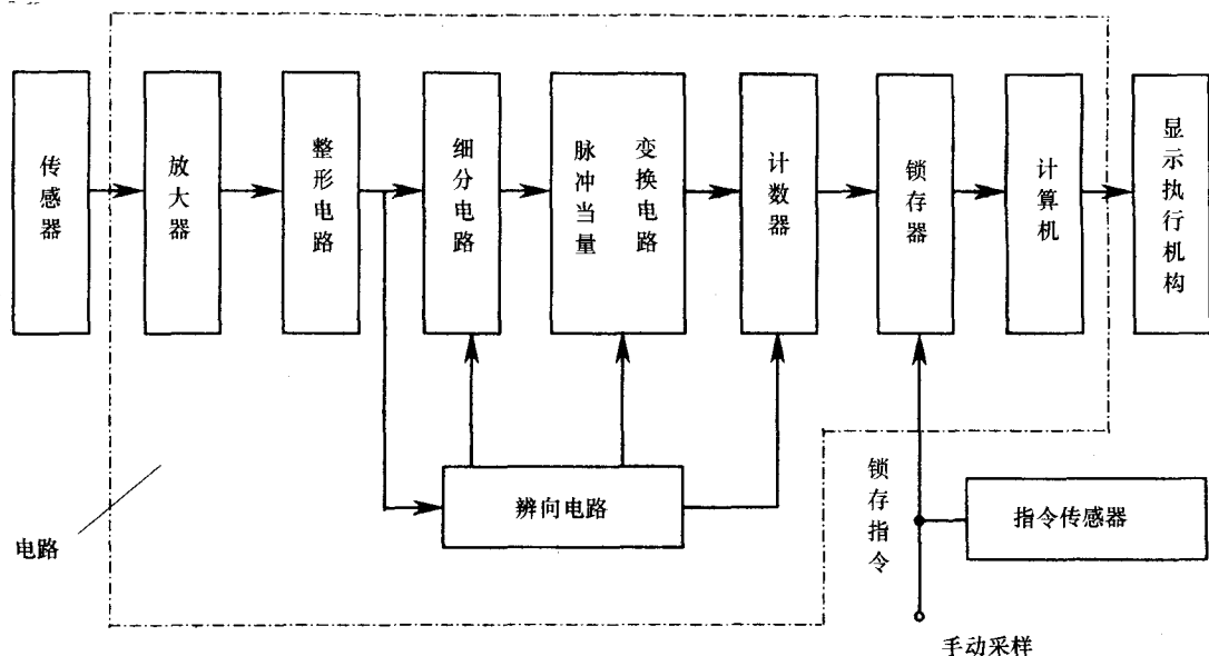
图 1-7 增量码数字式测量电路的基本组成
