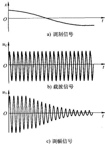
图 1-4 调幅信号
