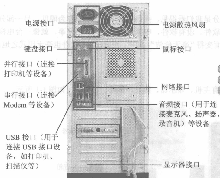
图 1-4 机箱的背面图
