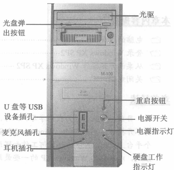
图 1-3 主机正面图
