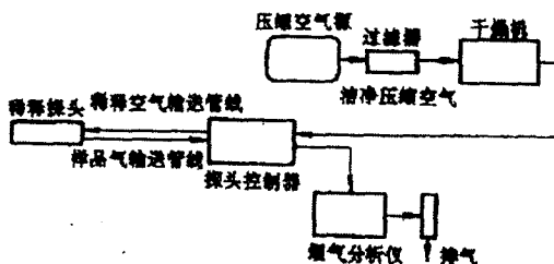
图 3 稀释抽取式烟气在线监测系统示意图
