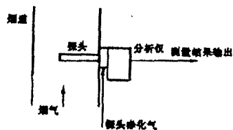
图 1 内置式烟气在线监测系统示意图
