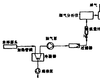
图 2 全抽取式烟气在线监测系统示意图
