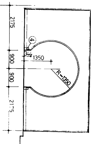
圆门洞立面
