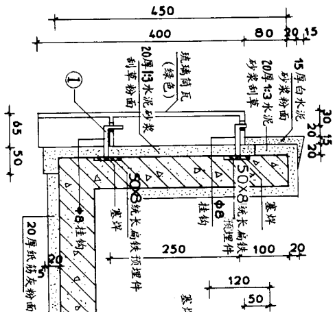
琉璃筒瓦檐口剖面详图
