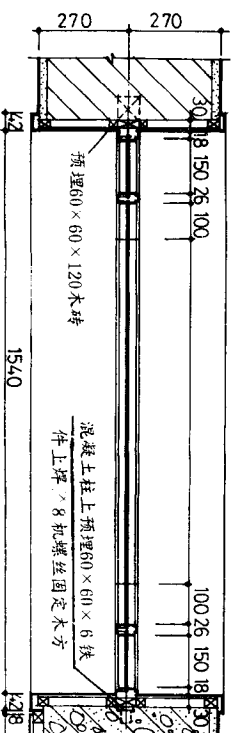
花窗平面
