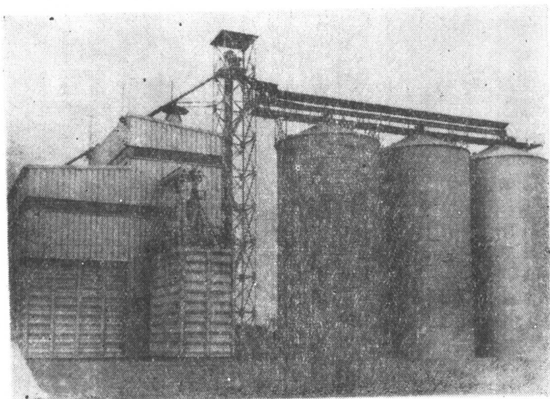
县饲料公 司饲料立筒仓
