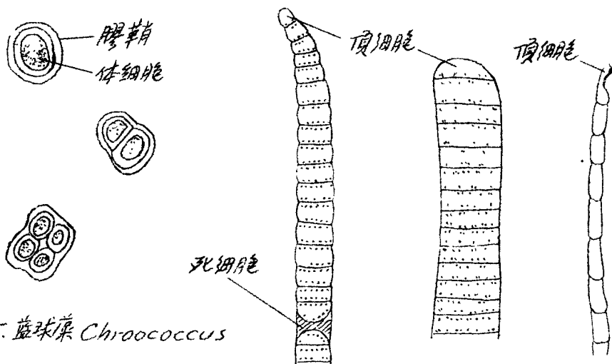
图26. 颤藻 Oscillatoria
