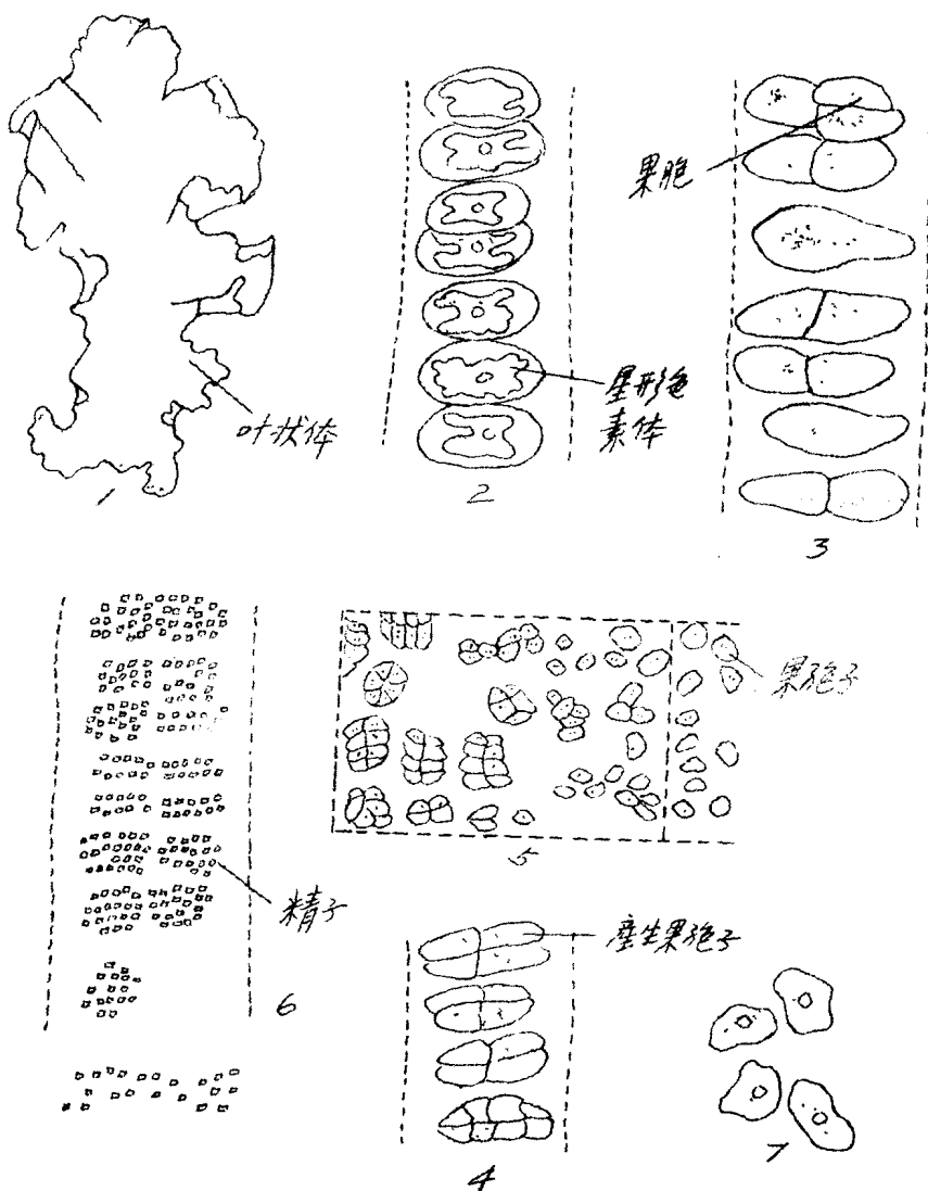
图23. 紫菜 Porphyra
