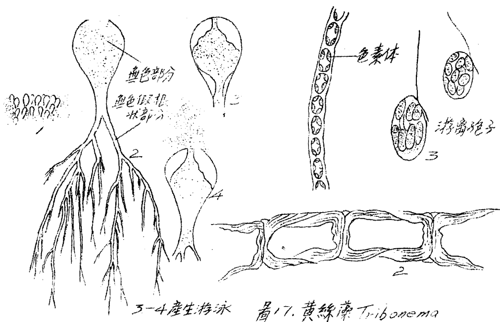
圖16. 氣球藻 Botrydium
