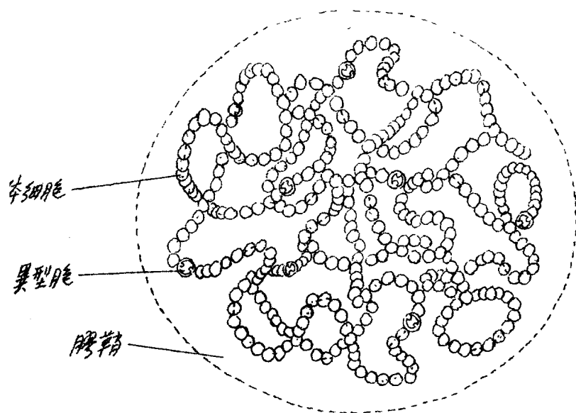
图27. 念球藻 Nostoc
