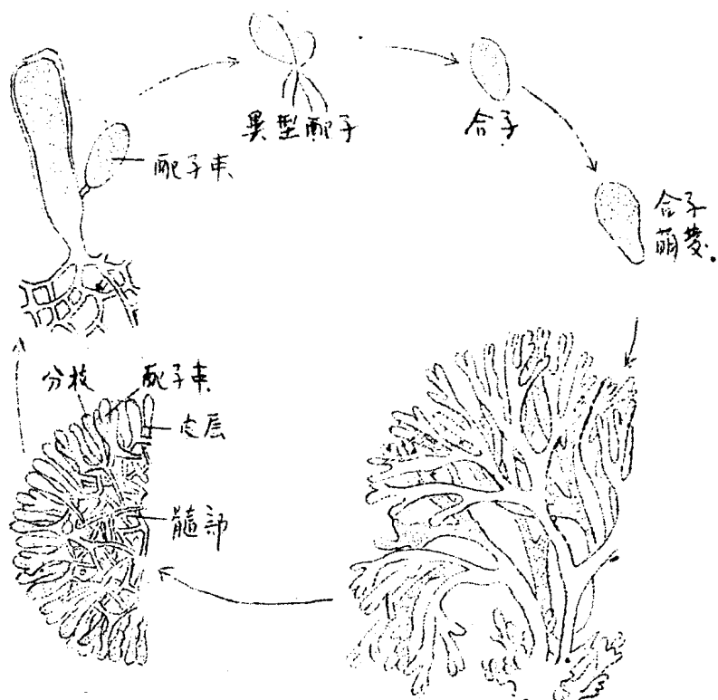
图12. 海松 Codium
