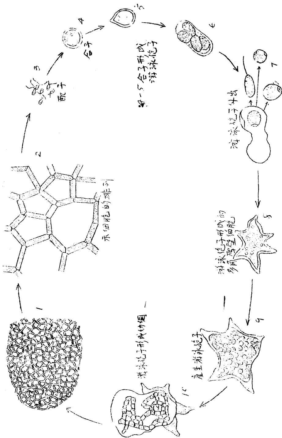
图 8. 水倮 Hydrodictyon
