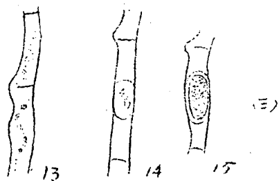
图13. 水绵 Spirogyra
