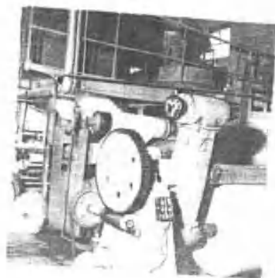
桥式涂布机机头及收纸部分
