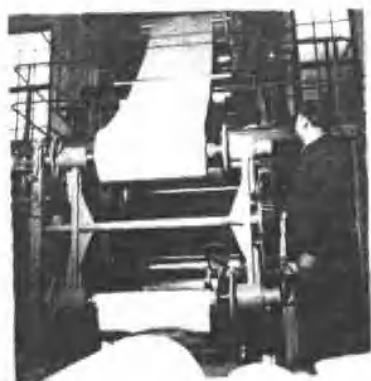
铜版纸七辊压光机正面
