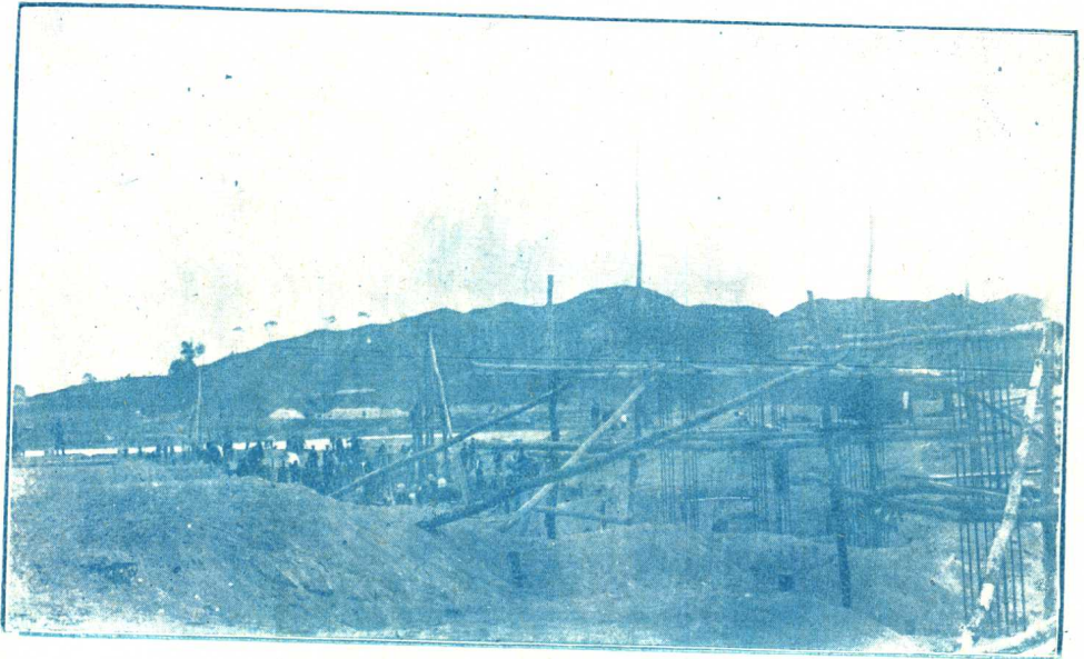
第九區信葉綾河橋施工情形
