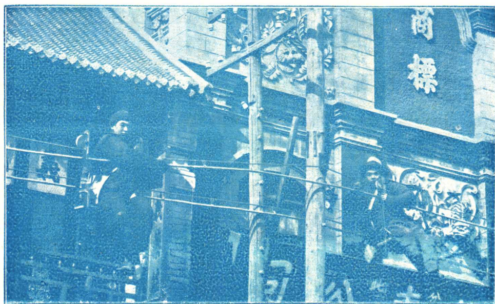
開 封 市 電 話 架 空 電 纜 安 裝 掛 鉤 情 形
