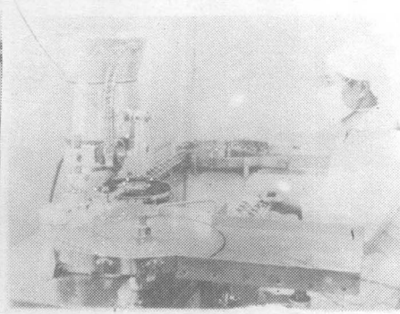
南京药械厂的自动分装半加塞流水线
