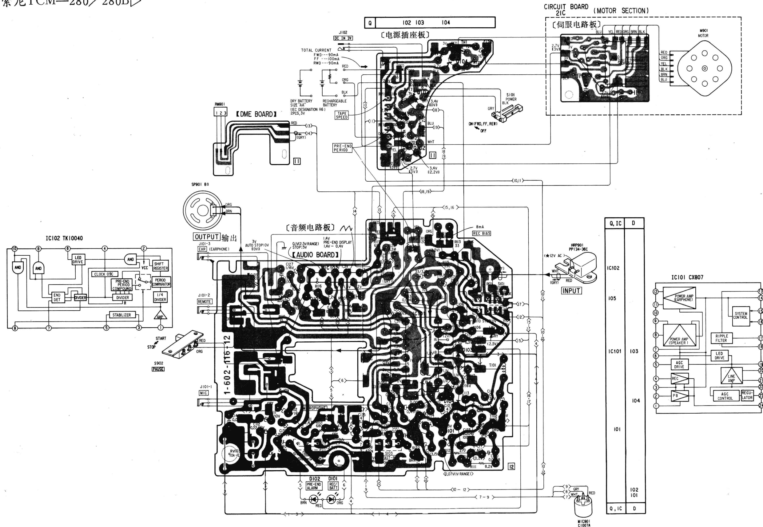
印刷电路图
