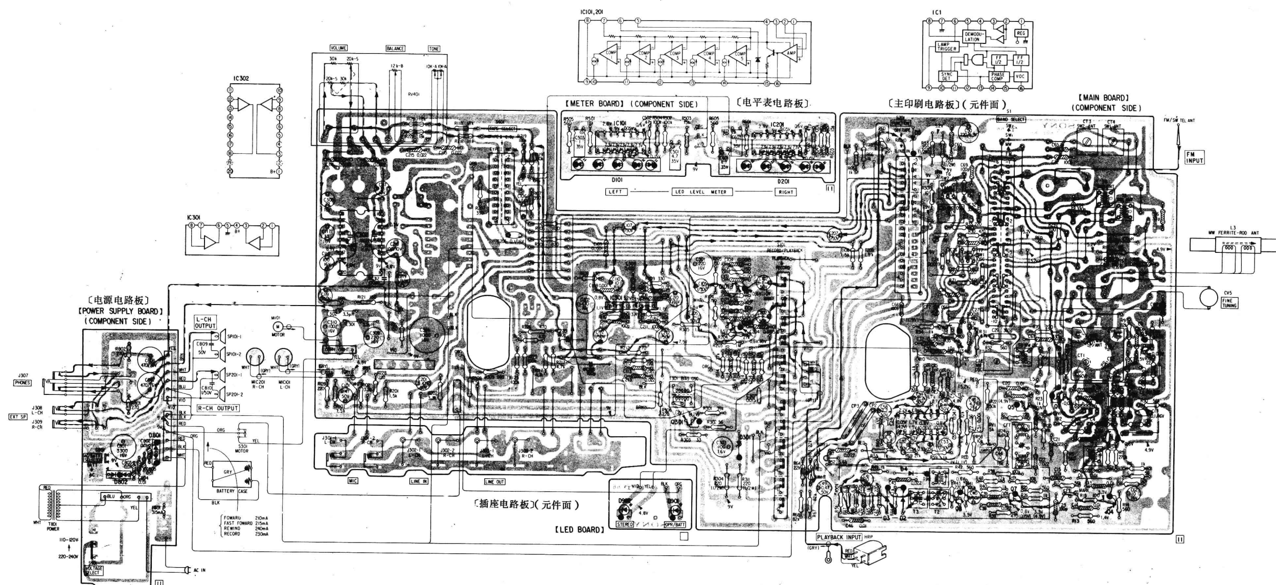
印刷电路图 (元件面)
