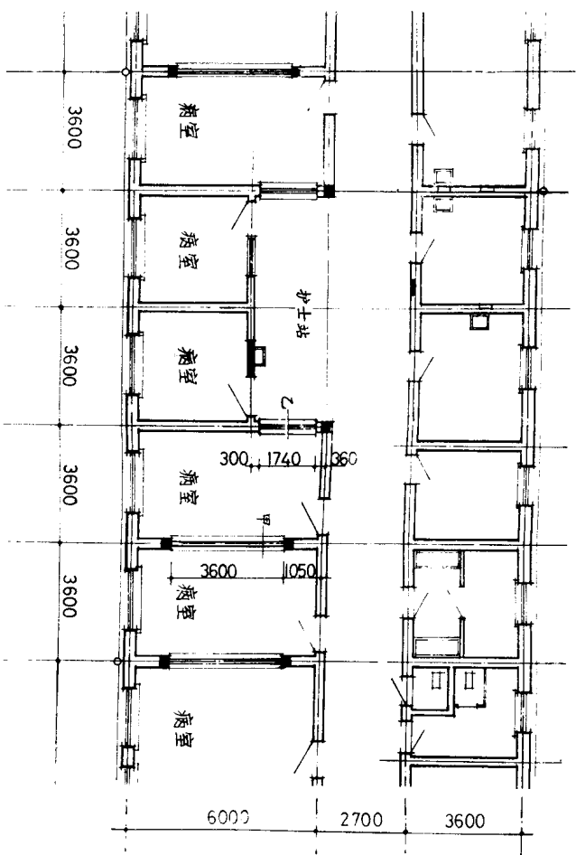
儿科病房局部平面
