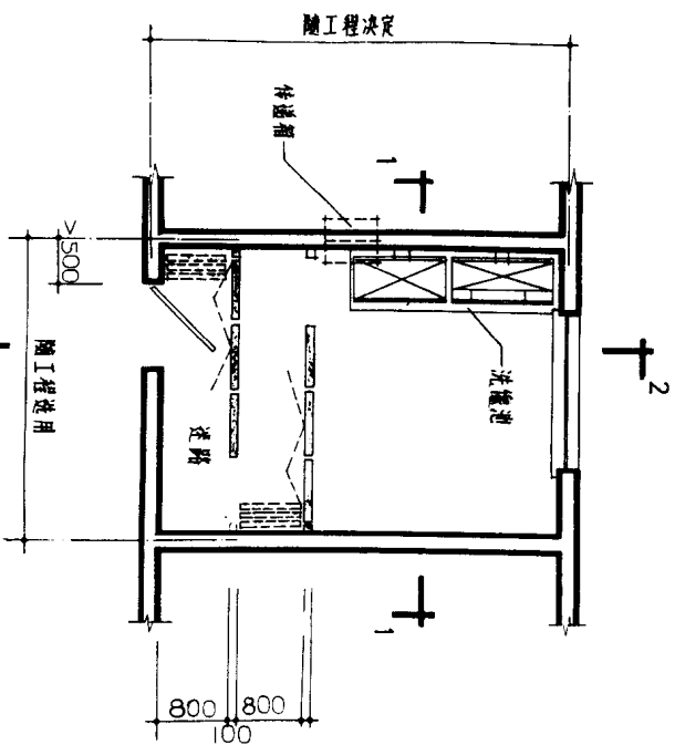
洗片室平面布置图
