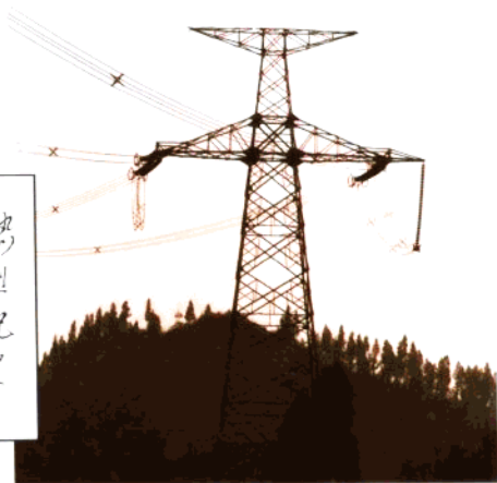
参建中国第一条±500kV 直流葛(洲坝)—上(海)输电线路工程(1987,部优)
