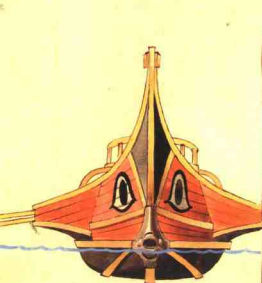
古希腊战船船尖及其剖面图
