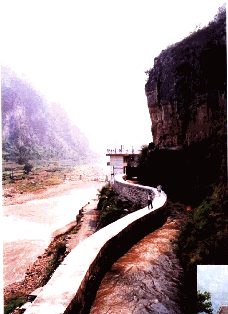
总干渠瓮枢纽间
