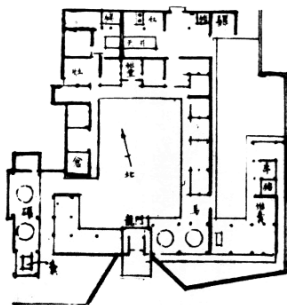
四川廣漢縣住宅平面圖(三)
