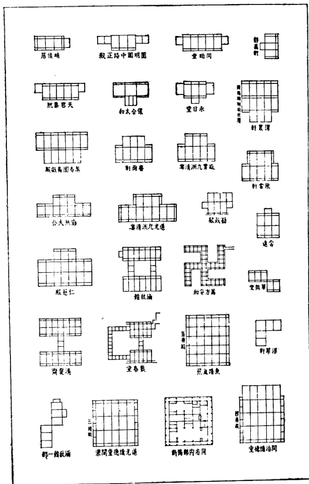
中國建築各種平面
