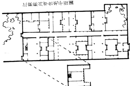
江蘇蘇州市住宅平面圖
