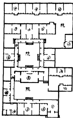
北京住宅平面圖(四)
