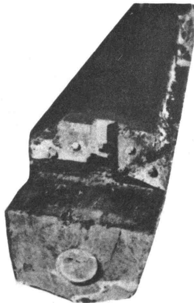
出土海船的保寿孔。(左)
