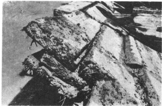
出土宋代海船的三层船板结构
