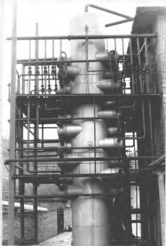
碳化塔
