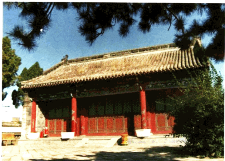
文庙大成殿
