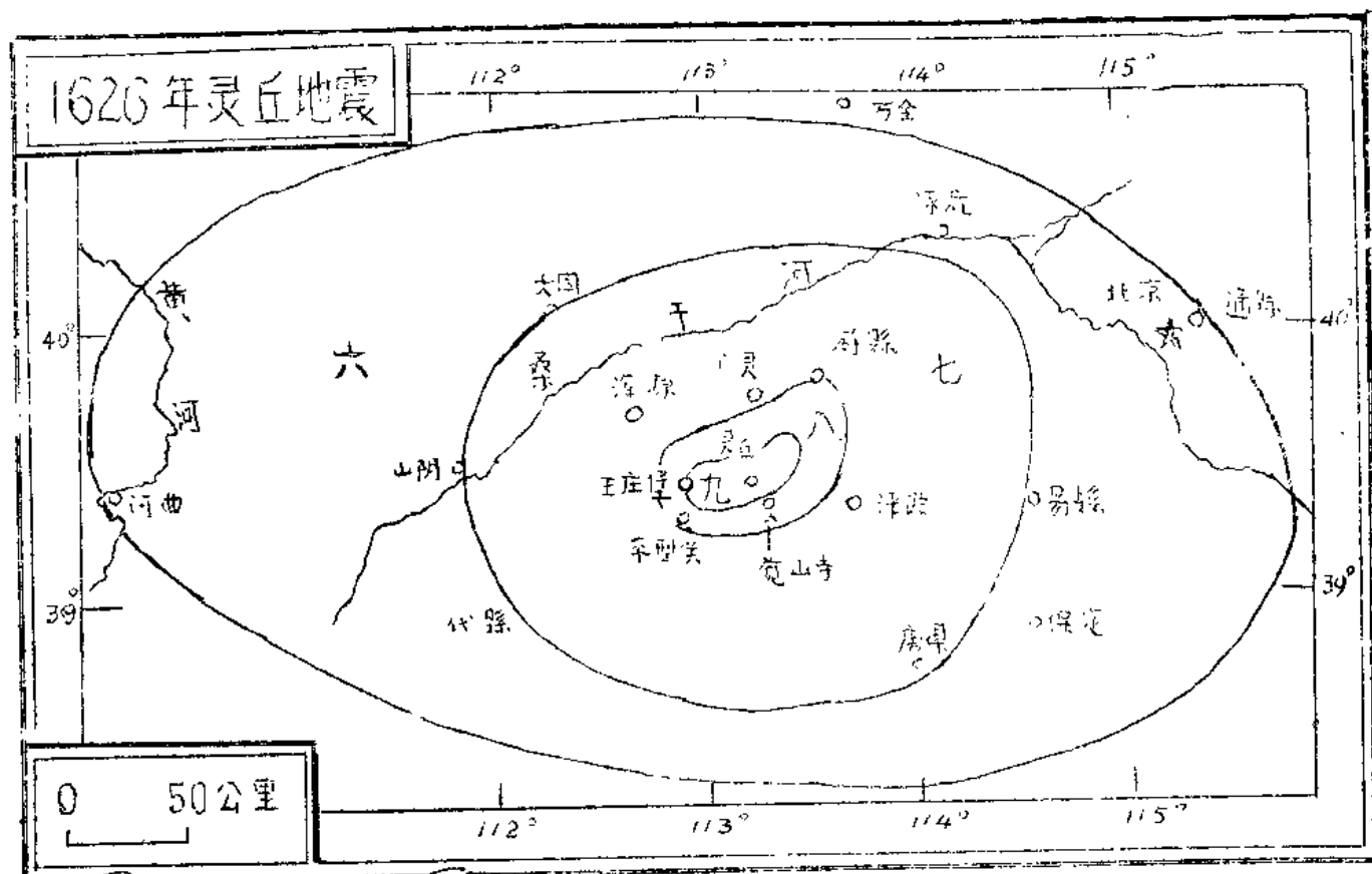
1626.6.28 山西灵丘地震等震线图
