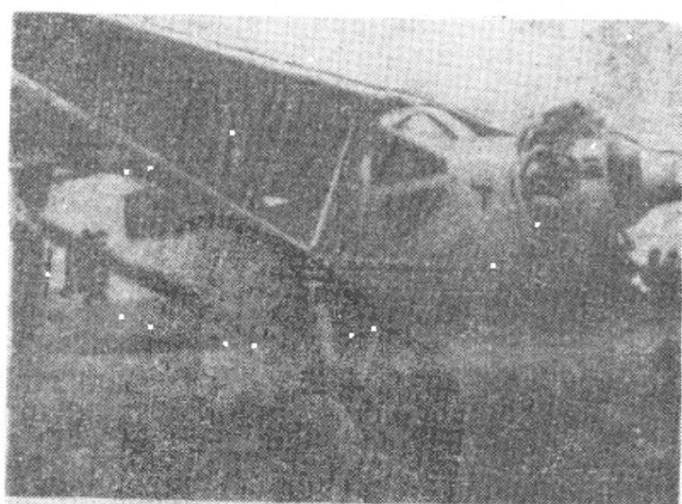
1928年11月11日中国第一次长途飞行使用的 “广州”号——瑞安NYP-2 (B-5) 陆上飞机
