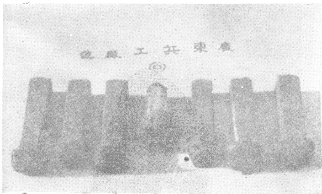
紫金县炮子兵工厂使用过的工具——钢戳。当年兵工厂制造的枪支都用这些钢戳打上“广东兵工厂造”的钢印
