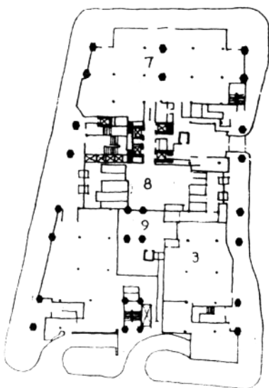
一层平面
