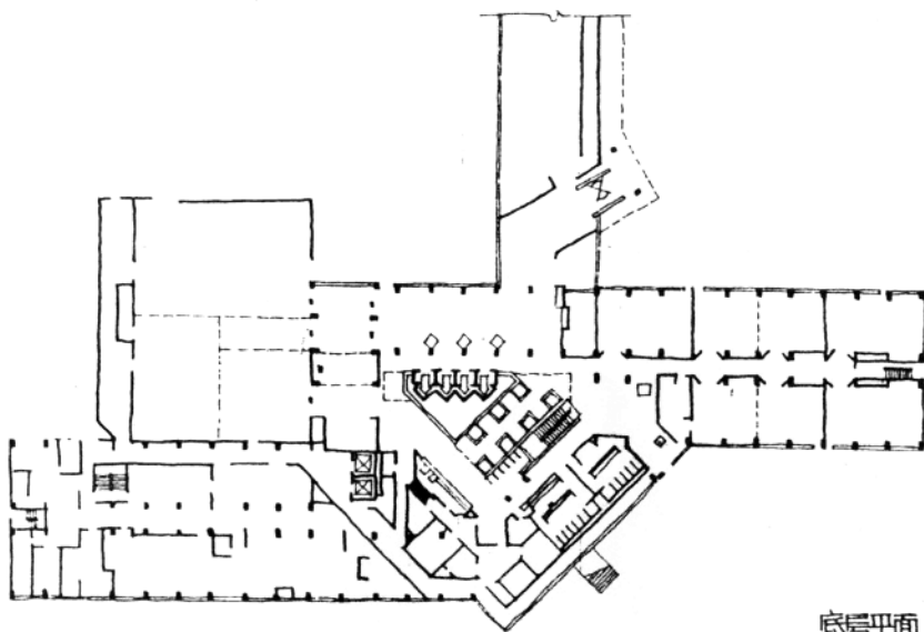
底层平面
