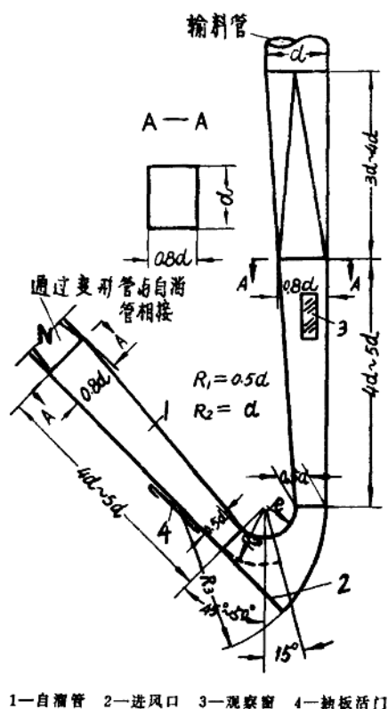
图 1-5 诱导式三通接料器
