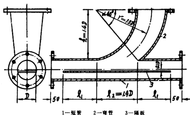
图 1-3 卧式三通接料器
