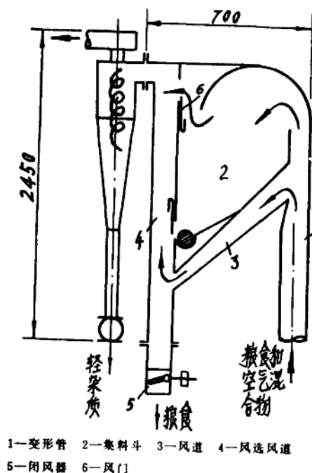
图 1-12 风动分离器
