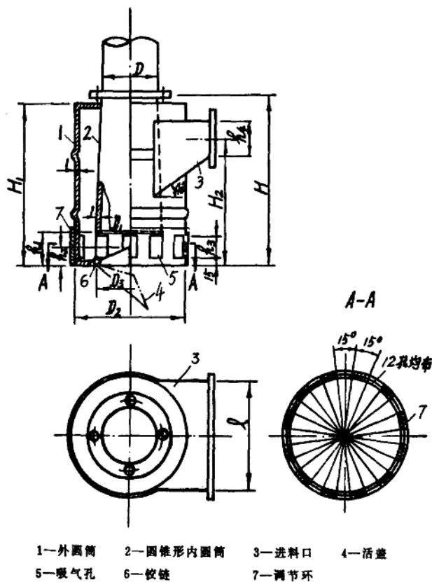
图 1-2 环吸式套筒接料器
