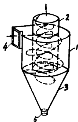
1—外圆筒 2—内圆筒 3—圆锥筒 4—进气口 5—排料口
