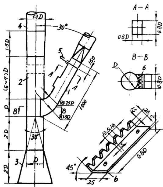
图 1-4 直立式三通接料器
