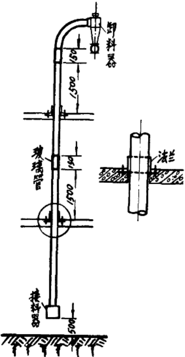
图 1-6 输料管安装示意图
