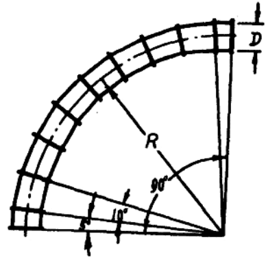
图 1-7 90°弯头
