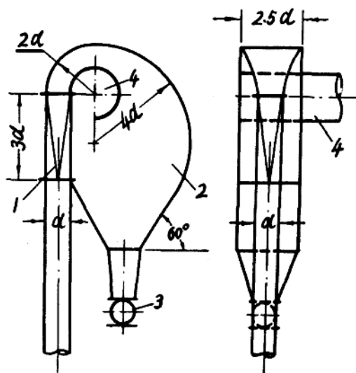
1—变形管 2—沉降室 3—闭风器 4—开口圆管
