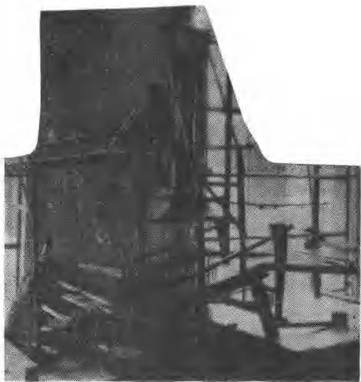
旧时成都织锦工人使用的“长机”（摄于四川省博物馆）
