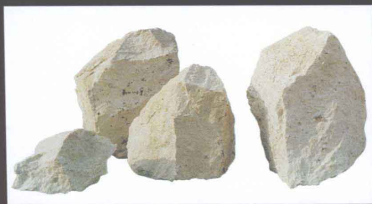
石英斑岩
