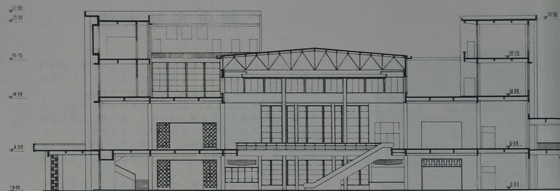
剖面图
