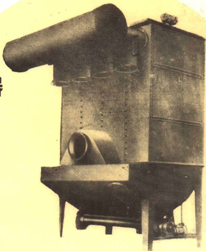
FD型反吹风袋式除尘器 曾荣获鞍山市科研三等奖
