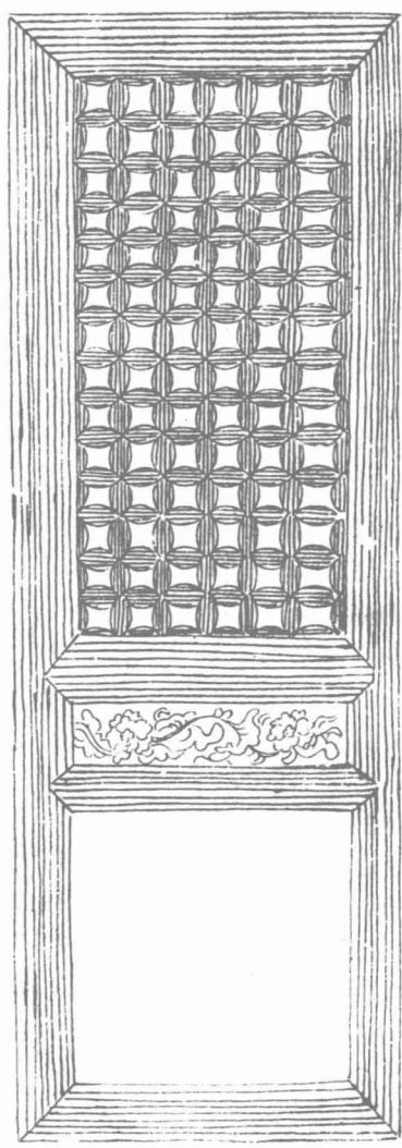
四直球文上出條枳重格眼 四枳四混出單線
