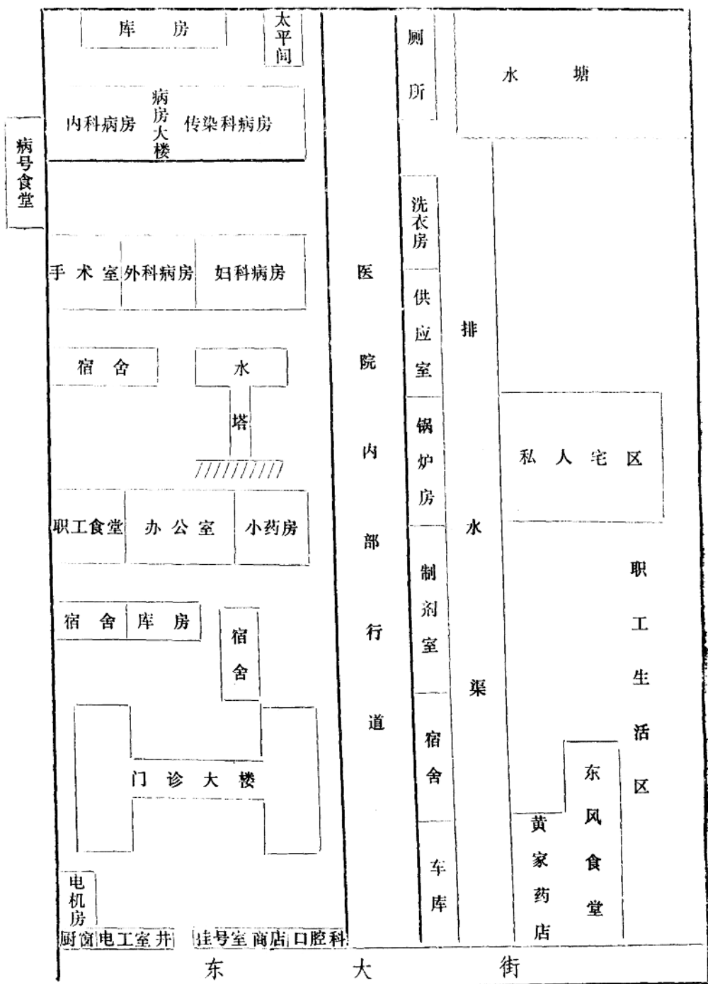
内黄县人民医院(1982)年平面图
