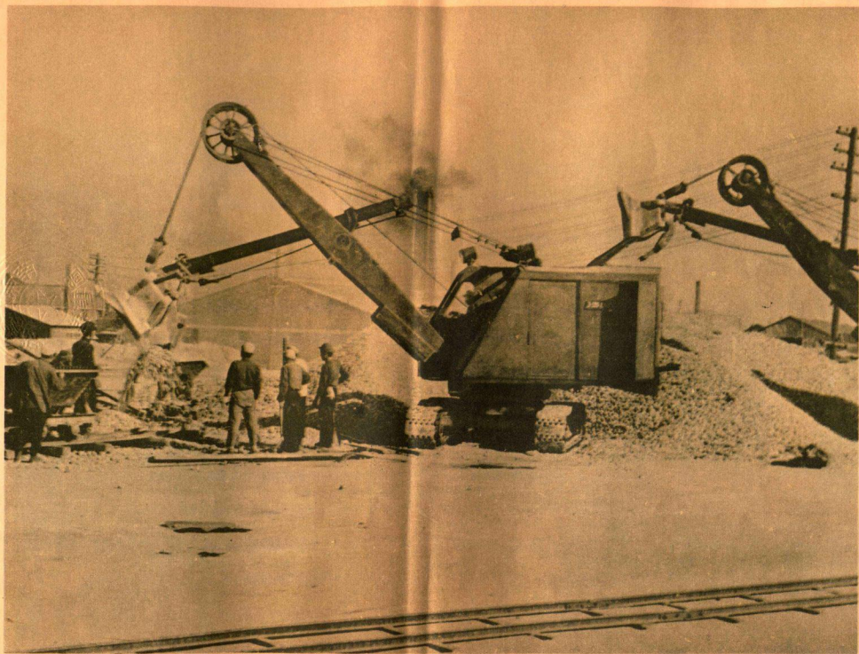
7 鞍鋼基本建設工程中使用的石塊、石子全部是用機器裝載的。圖中即為機器裝載石塊、石子的情形。
