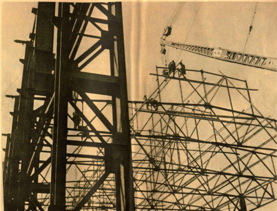
13 鞍鋼基本建設工程中的架工們正以靈敏而又熟練的技術在從事高空作業。
