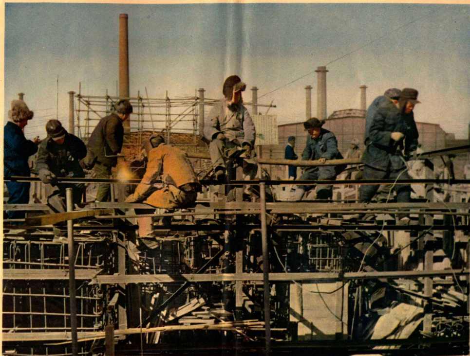
11 鞍鋼的基本建設規模是空前巨大的。其中如某工程的一個基礎，就要挖掘土方七千四百多立方公尺，需要鋼筋和附屬零件二百三十五噸。這樣巨大的基礎工程必須由鋼筋、混凝土和管道等工人充分合作才能順利完成。這是鋼筋工人在基礎工程上從事鋼筋綁紮工作時的情形。
