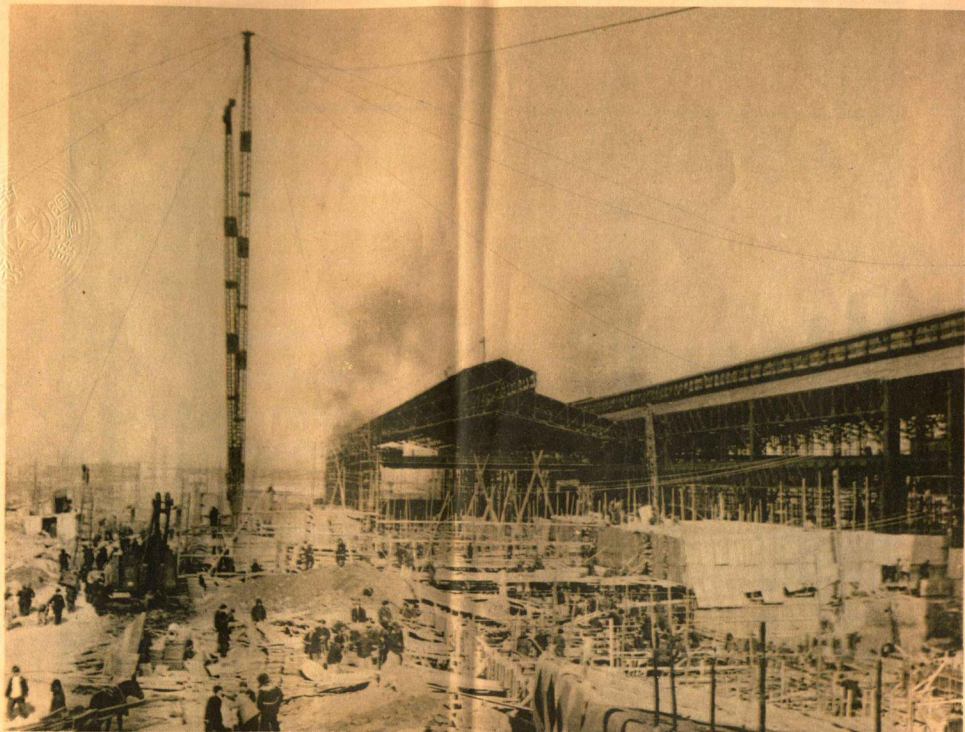
8 鞍山基本建設工程中大量的吸收蘇聯的先進經驗，在加速重大工程的進度與保證工程的質量上具有決定性的作用。圖中有席篷的地方是採用蘇聯先進的工作方法，進行冬季施工的保溫設備。由於冬季施工，一年可以增加三四個月的作業時間。
