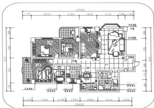
01 平面图
