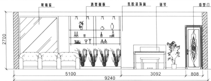
02 立面图1
