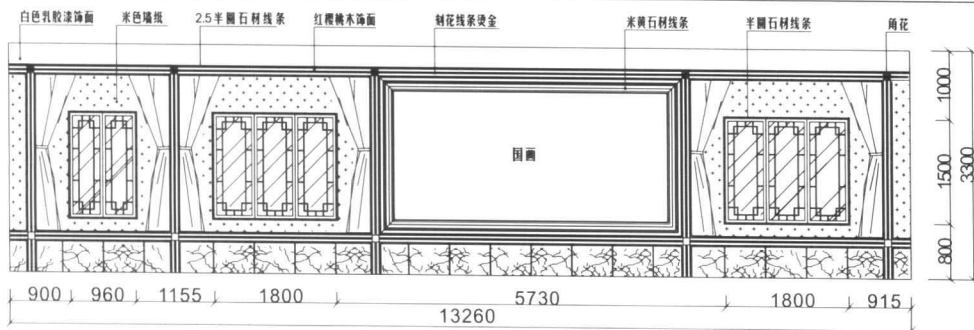
03 立面图2
