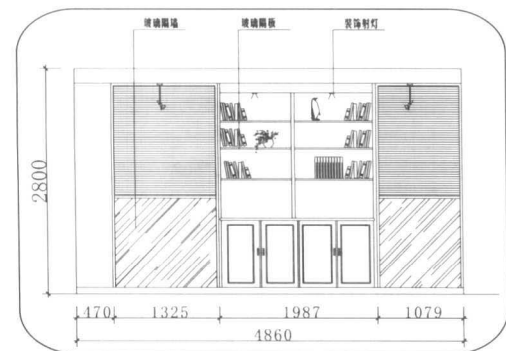
04 书柜立面图
