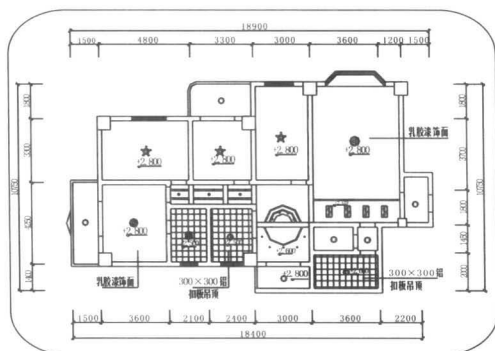
02 天棚图
