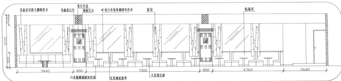
02 立面图1
