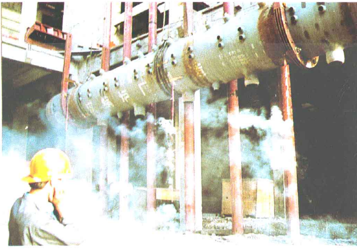
一号炉汽包起吊
