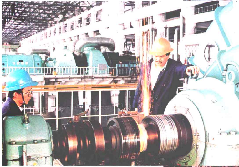
发电机滑环磨削新工艺
