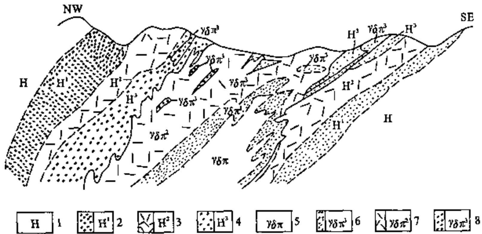
图 II-3 铜厂矿床蚀变分带剖面略图
