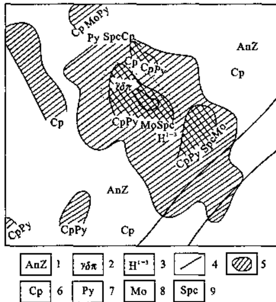
图 II-4 德兴斑岩铜矿田重砂异常略图
