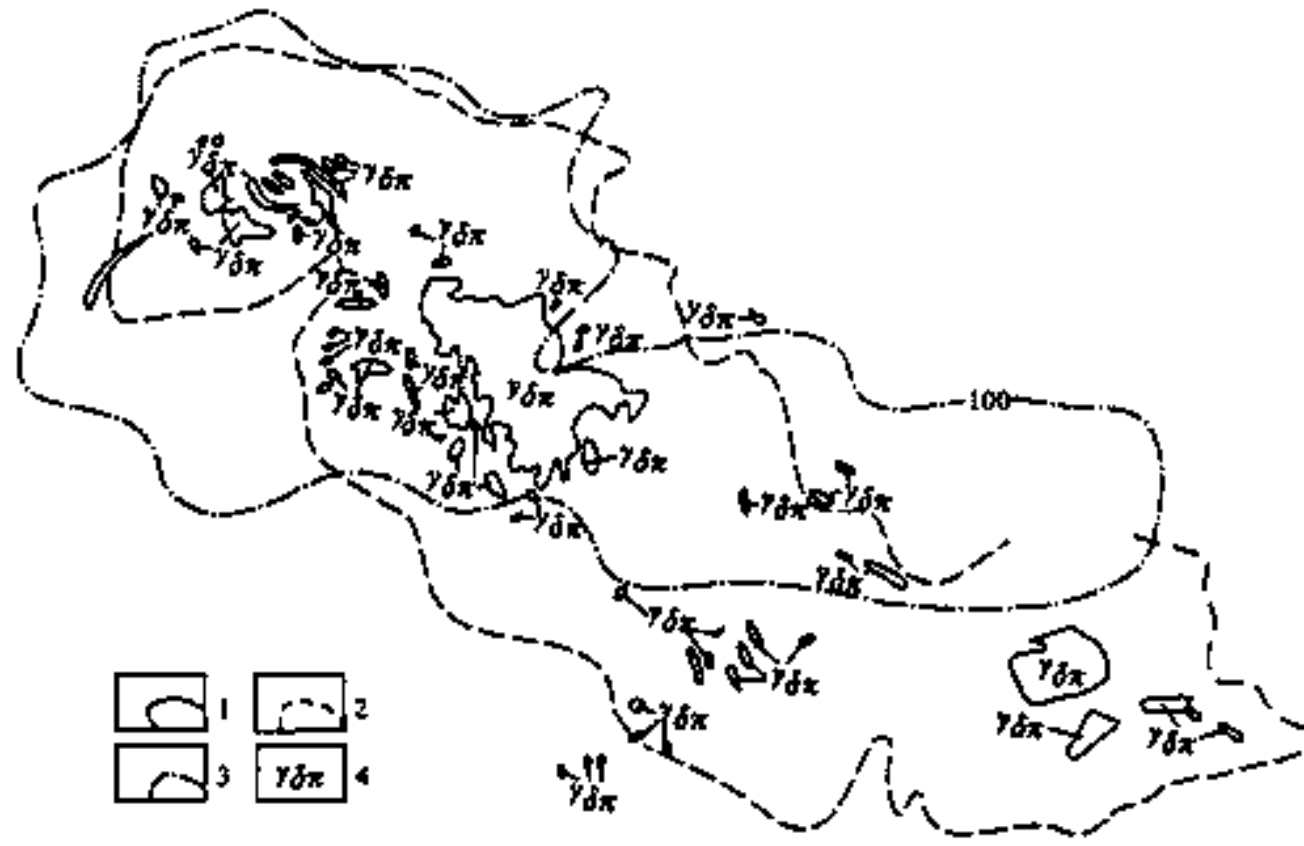
图 II-7 矿田地磁 \Delta Z 异常图
