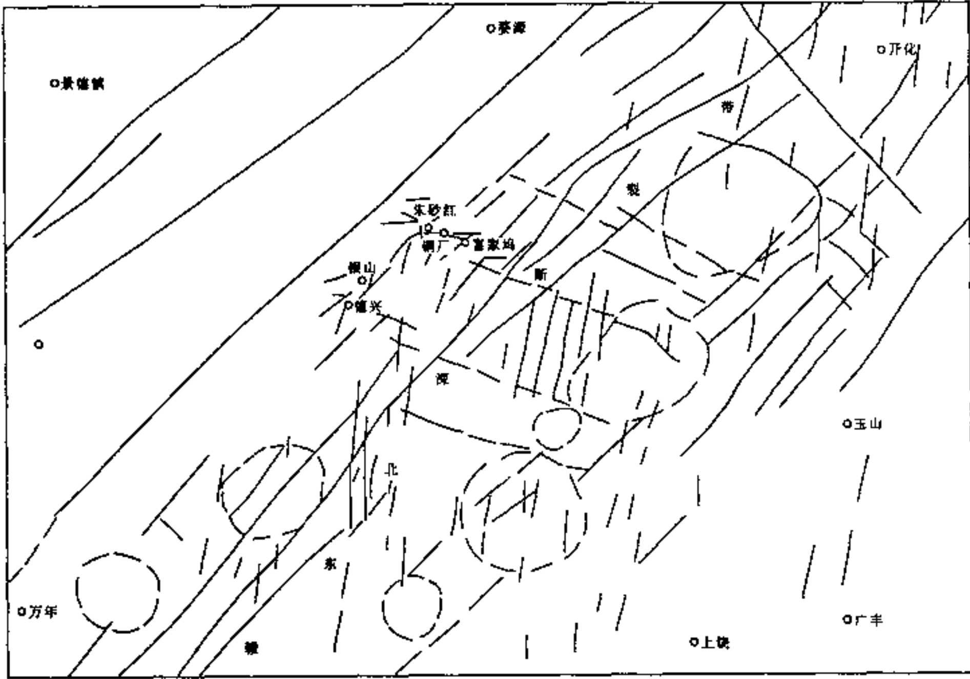
图 II-2 赣东北深断裂带卫星照片解译图
