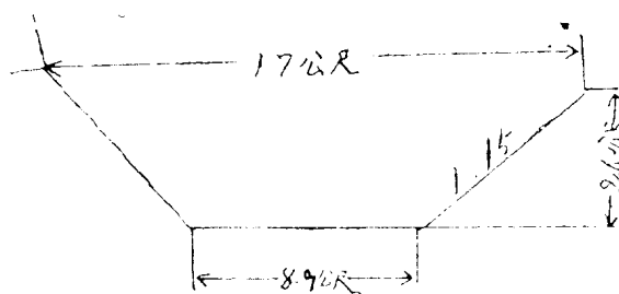
下游橫断面圖
