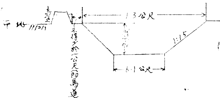
上游橫断面圖
