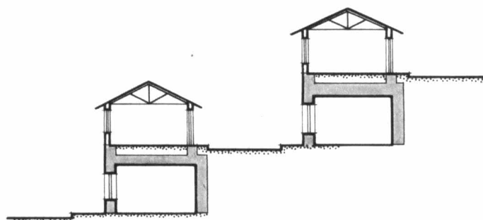
窑洞剖面图
