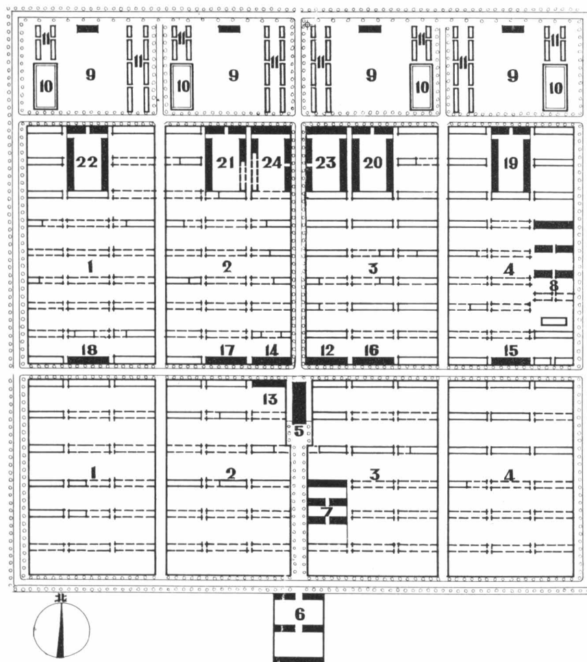
后屯大队新村总平面图
