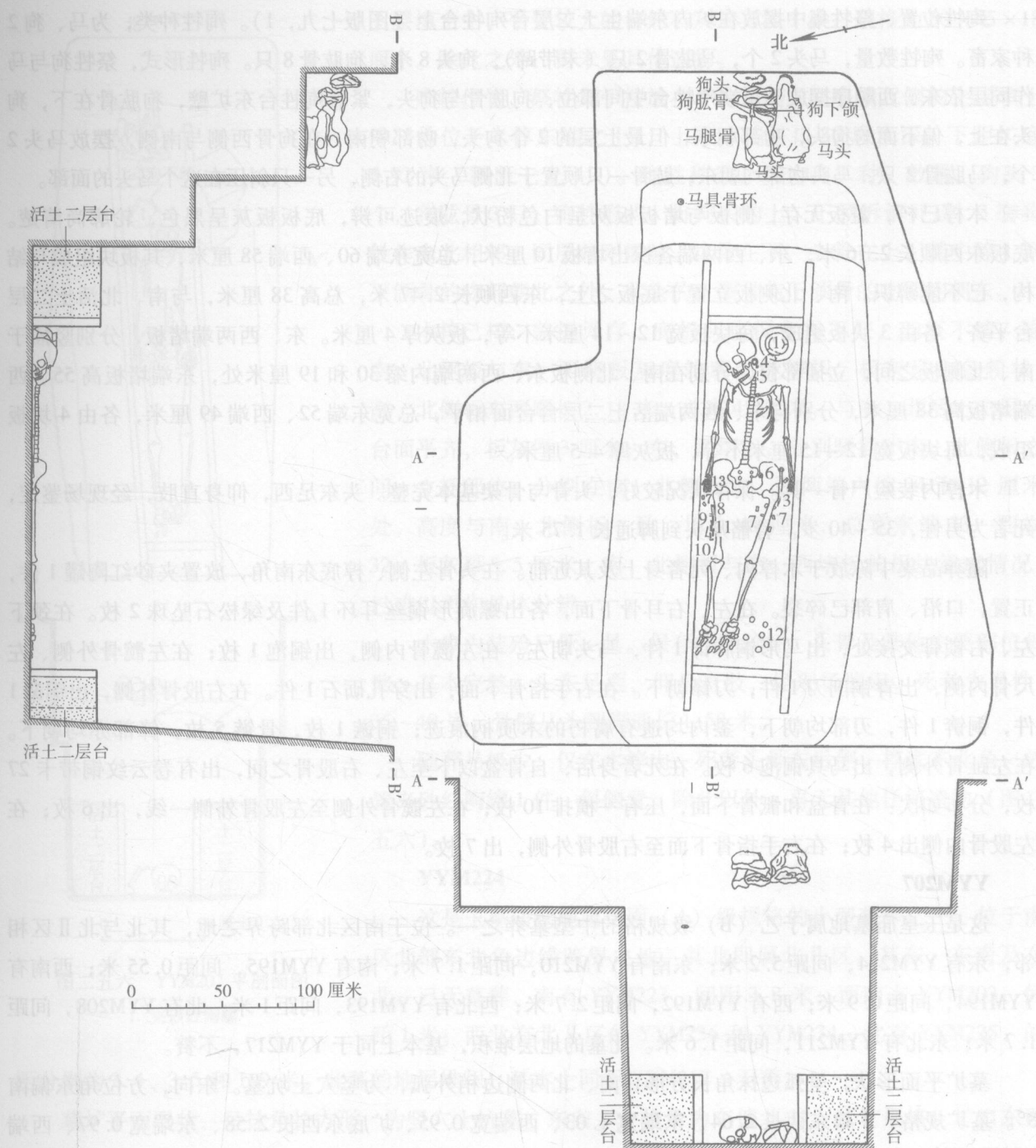
图二五五 YYM217 平剖面图
