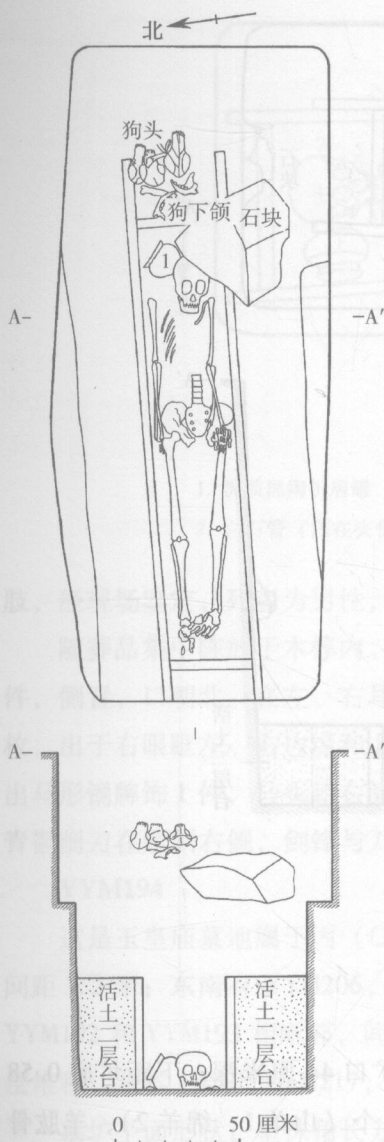
图二五六 YYM207 平剖面图
