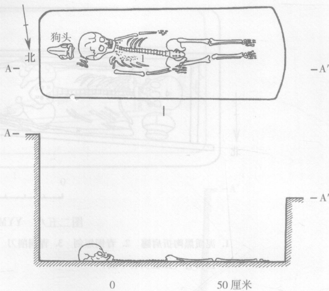
图二五九 YYM194 平剖面图
