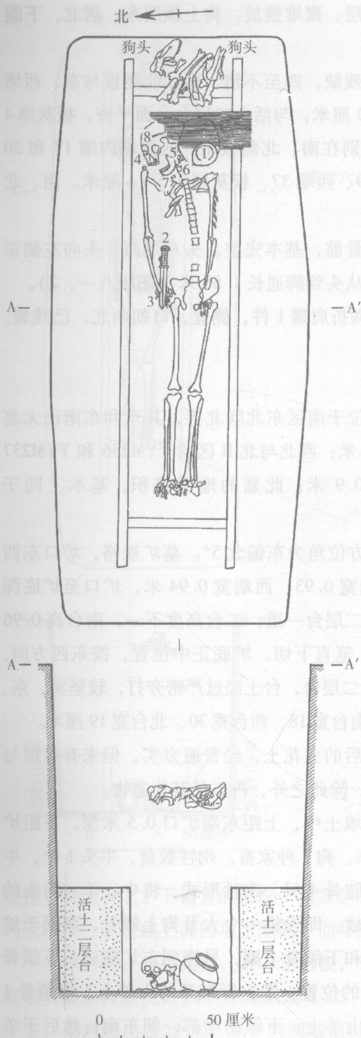
图二六〇 YYM182 平剖面图
