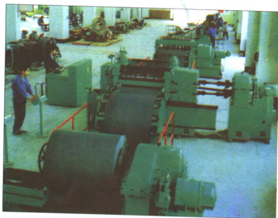
铁芯片纵向剪切线
