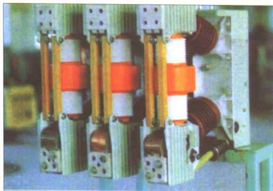
ZN12—10型真空断路器(德国西门子技术)
