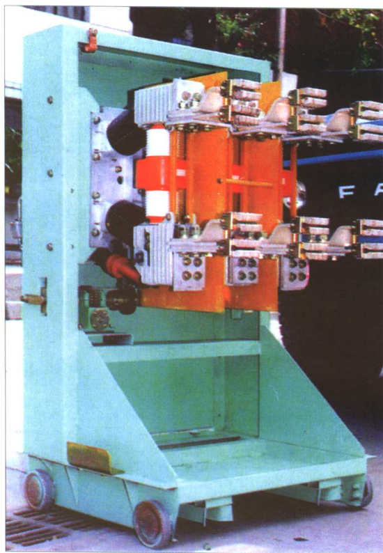
GFC—3BD型高压移开式开关柜内装3000A油断路器改装为ZN12—10、3150A(31.5KA、40KA、50KA)真空断路器(德国西门子技术)。
