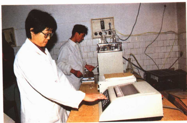
高效液相色谱仪
