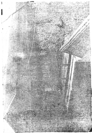
岱河咀扬水站： 在大名县城南偏东七公里处处卫河之北岸，此处是两水入卫之所，形似茶壶咀，也称岱河咀，故名。该站建于1973年，有八台机组，排涝流量为169立方米/秒，扬排流量为5立方米/秒。
