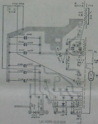
飞跃 9DS4 高压包板
