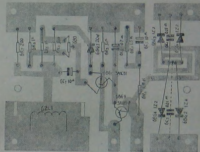
凯歌 4D4-A 电源板
