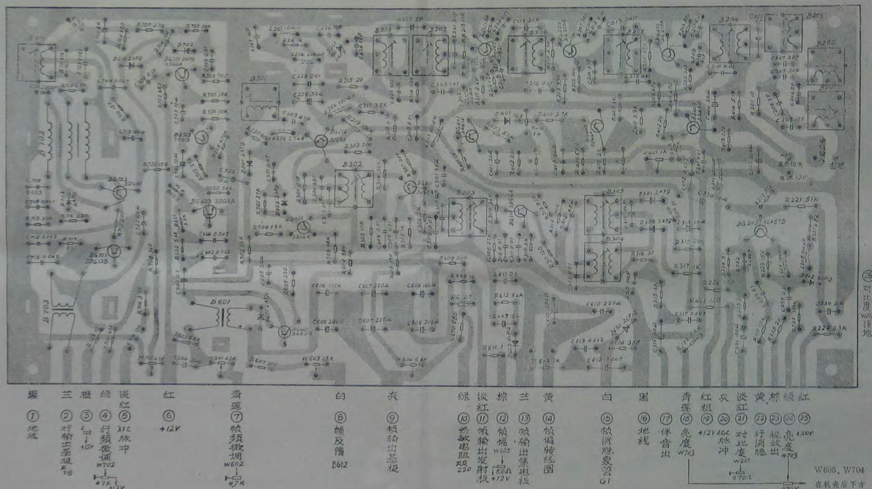
英雄 228-2 通道扫描板
