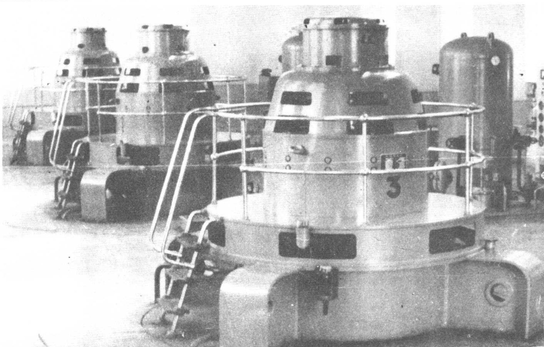
红山嘴电厂三级电站内景
