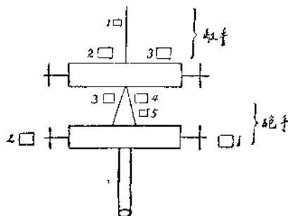
C 制退鋤翻上時之關係位置圖
