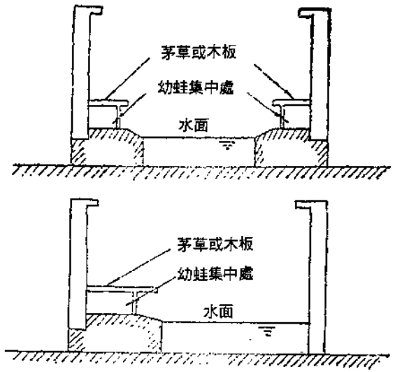
圖2 牛蛙親蛙池
